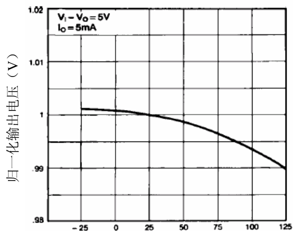
结温 (°C)
