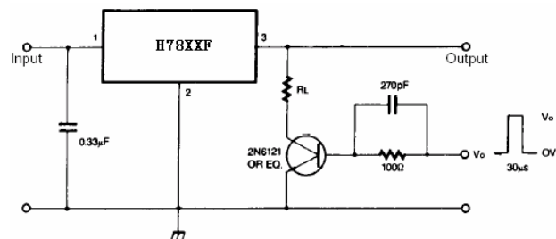
图 2、负载调整率测试
