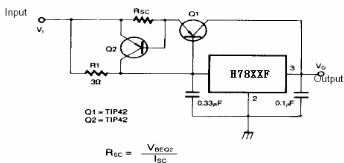
图 9、带短路保护的大电流输出
