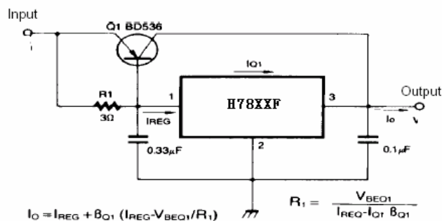
图 8、大电流稳压器
