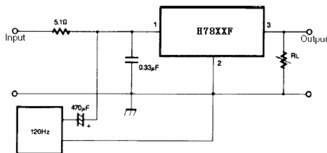
图 3、纹波抑制比测试
