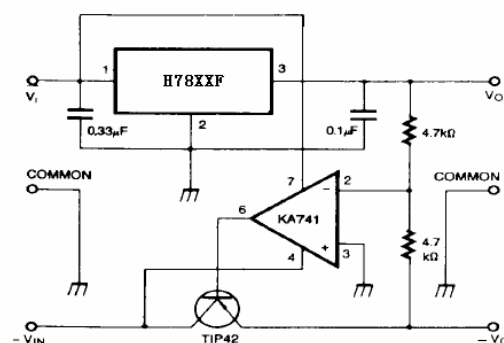
图 8、大电流稳压器
