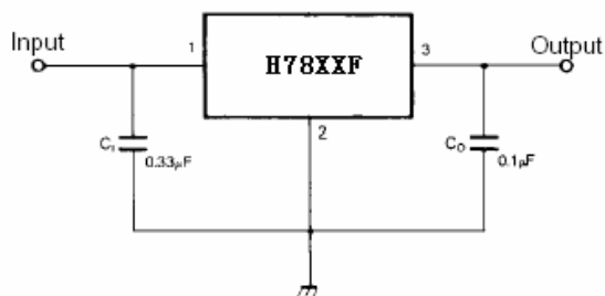
图 4、固定输出稳压器
