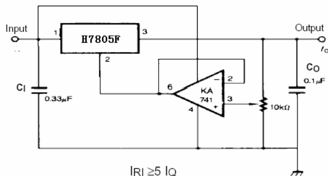
图 7、可调整输出稳压器(7~30V)
